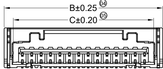
06P-15P Double Hole Scale 1:1
